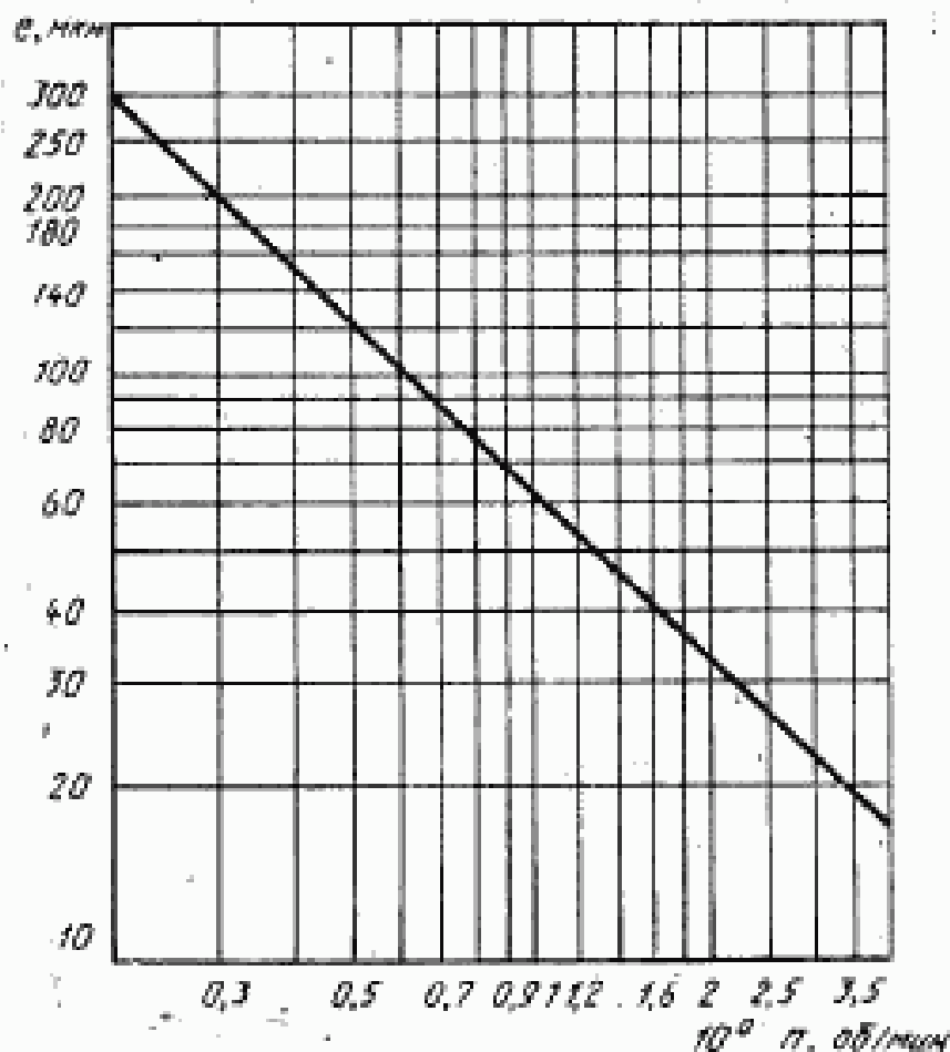
Допустимые удельные остаточные неуравновешенности рабочих колес вентиляторов
