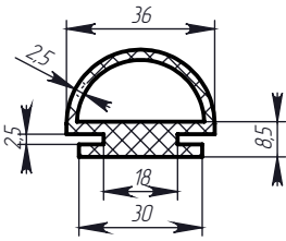
Профиль № 1114
