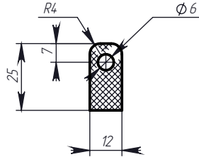
Профиль № 103
