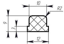
Профиль № 1125
