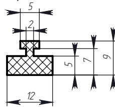
Профиль № 99
