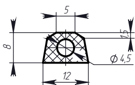
Профиль № 473
