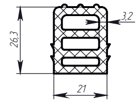
Профиль № 946
