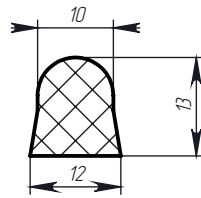
Профиль № 745
